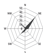
Průměrná četnost směrů větrů (%) za období 17. 5. - 19. 6. 2012
