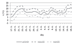
Chod průměrných teplot vzduchu (°C) v období 17. 5. - 19. 6. 2012
