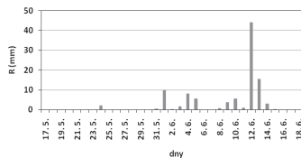
Průměrný denní úhrn srážek (mm) za období 17. 5. - 19. 6. 2012
