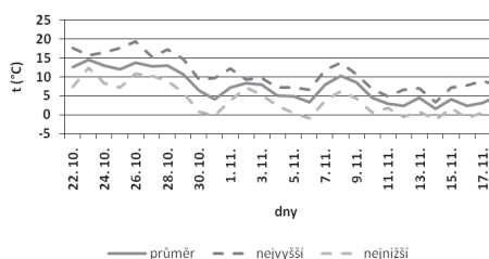
Chod průměrných teplot vzduchu (°C) v období 22. 10. - 18. 11. 2013
