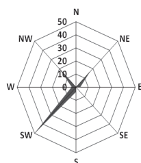
Průměrná četnost směrů větrů (%) za období 22. 10. - 18. 11. 2013
